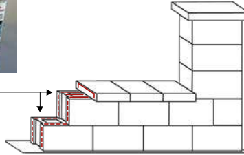
3. Füllbeton Menge des Anmachwassers laut Gebrauchsanweisung – zuviel Wasser mindert die Betonqualität. Wichtig: Füllbeton während der 28-tägigen Aushärtung vor Regen schützen!
